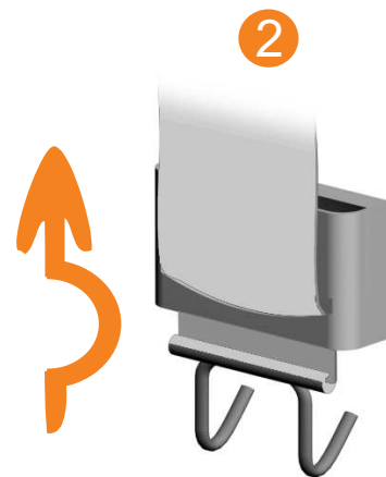
Passage/Montage sangle simple
